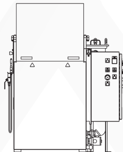
RTW-25
